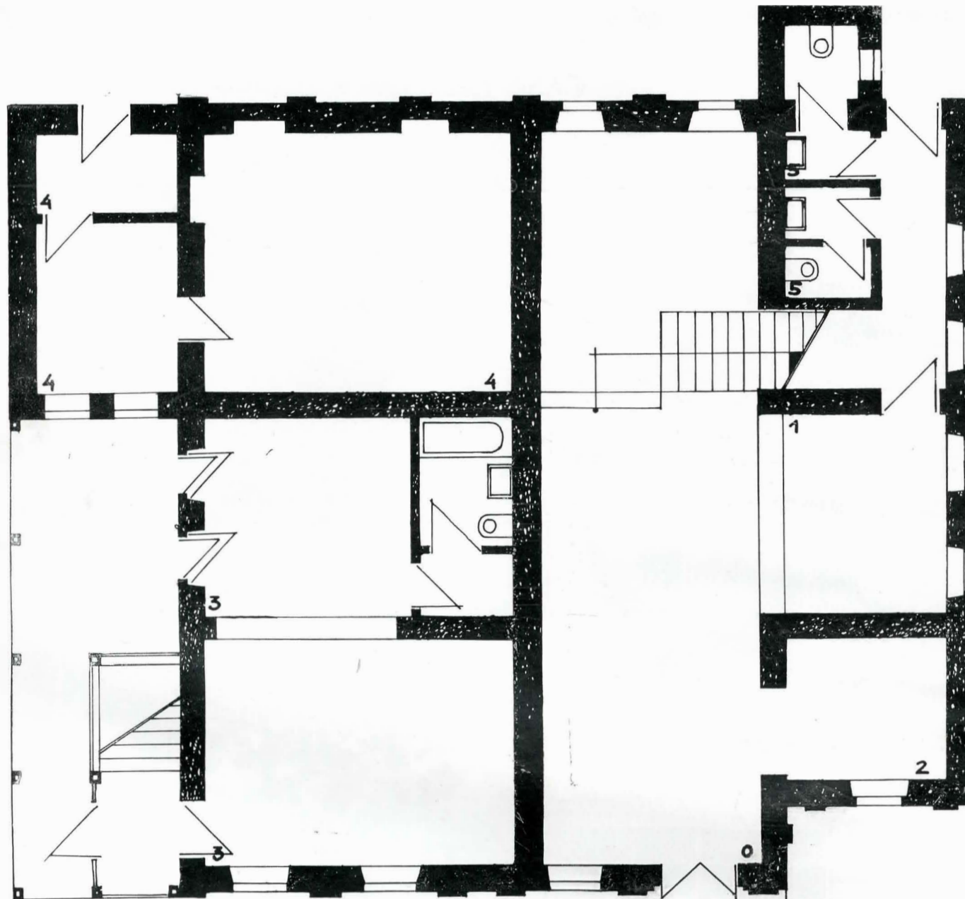
Fig. 2. Planul parterului: o - hol; 1 - muzeu (expunere); 2 - vestiar; 3 - apartamentul donatorului; 4 - anexe (spații de serviciu); 5 - grup sanitar public; 6 - debara.
